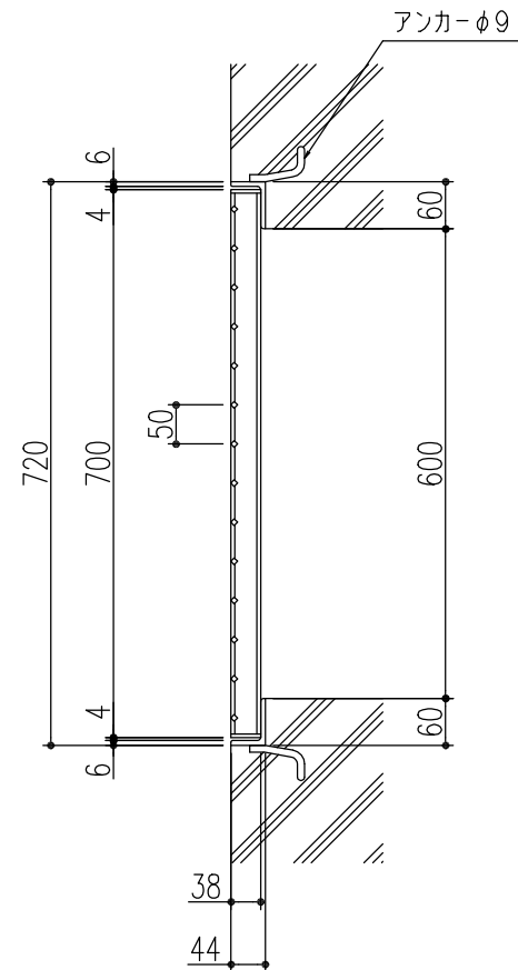
ベアリングバー 詳細図
