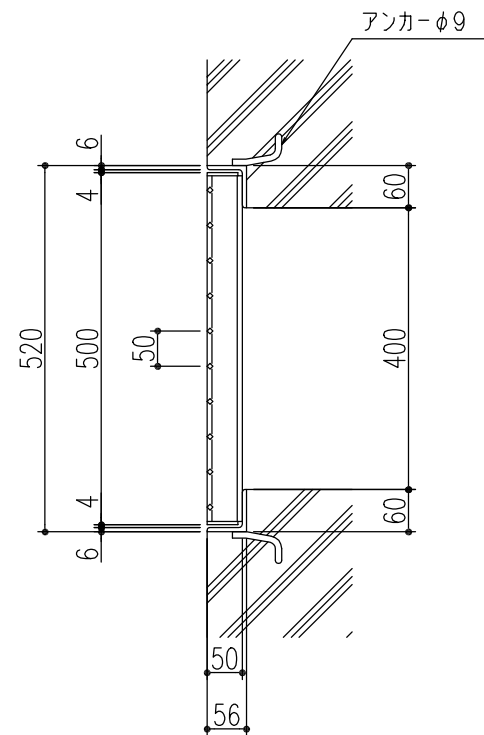
ベアリングバー 詳細図
