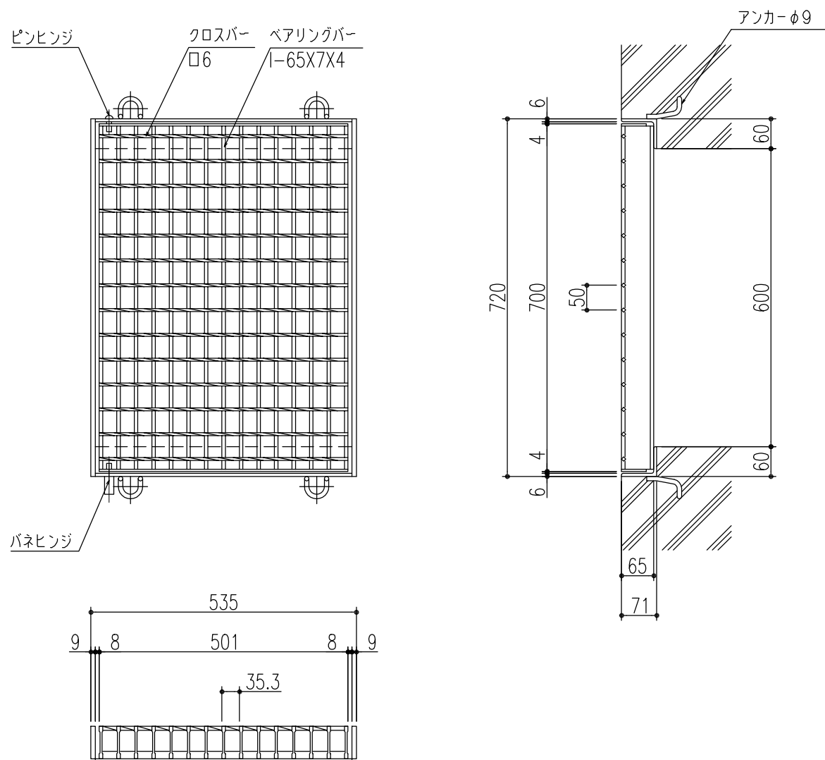
ベアリングバー 詳細図
