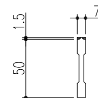
ベアリングバー 詳細図
