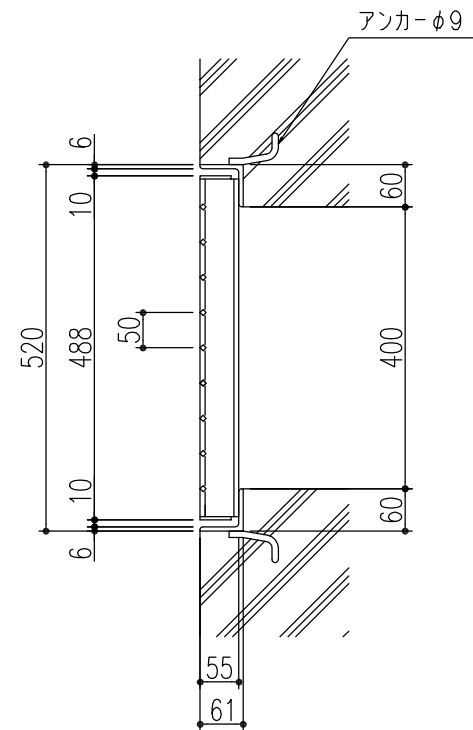
ベアリングバー 詳細図
