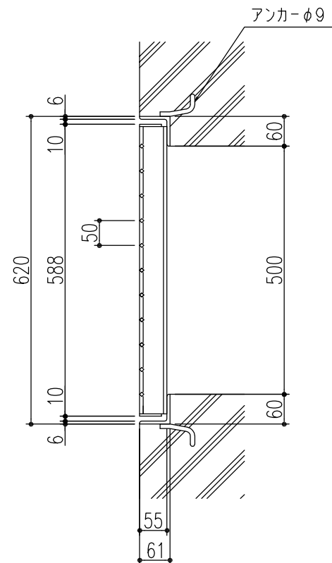
ベアリングバー 詳細図
