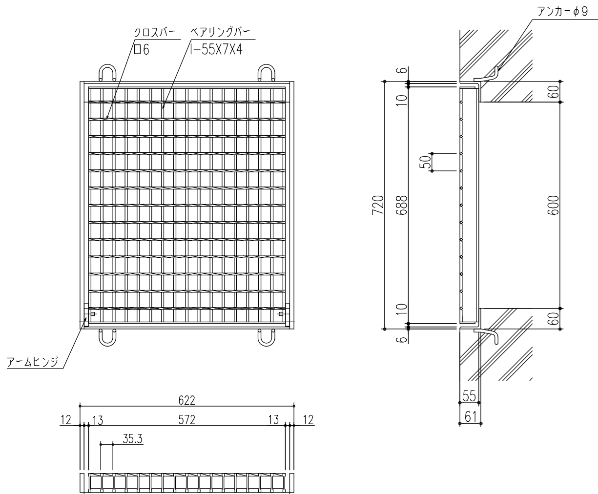
ベアリングバー 詳細図
