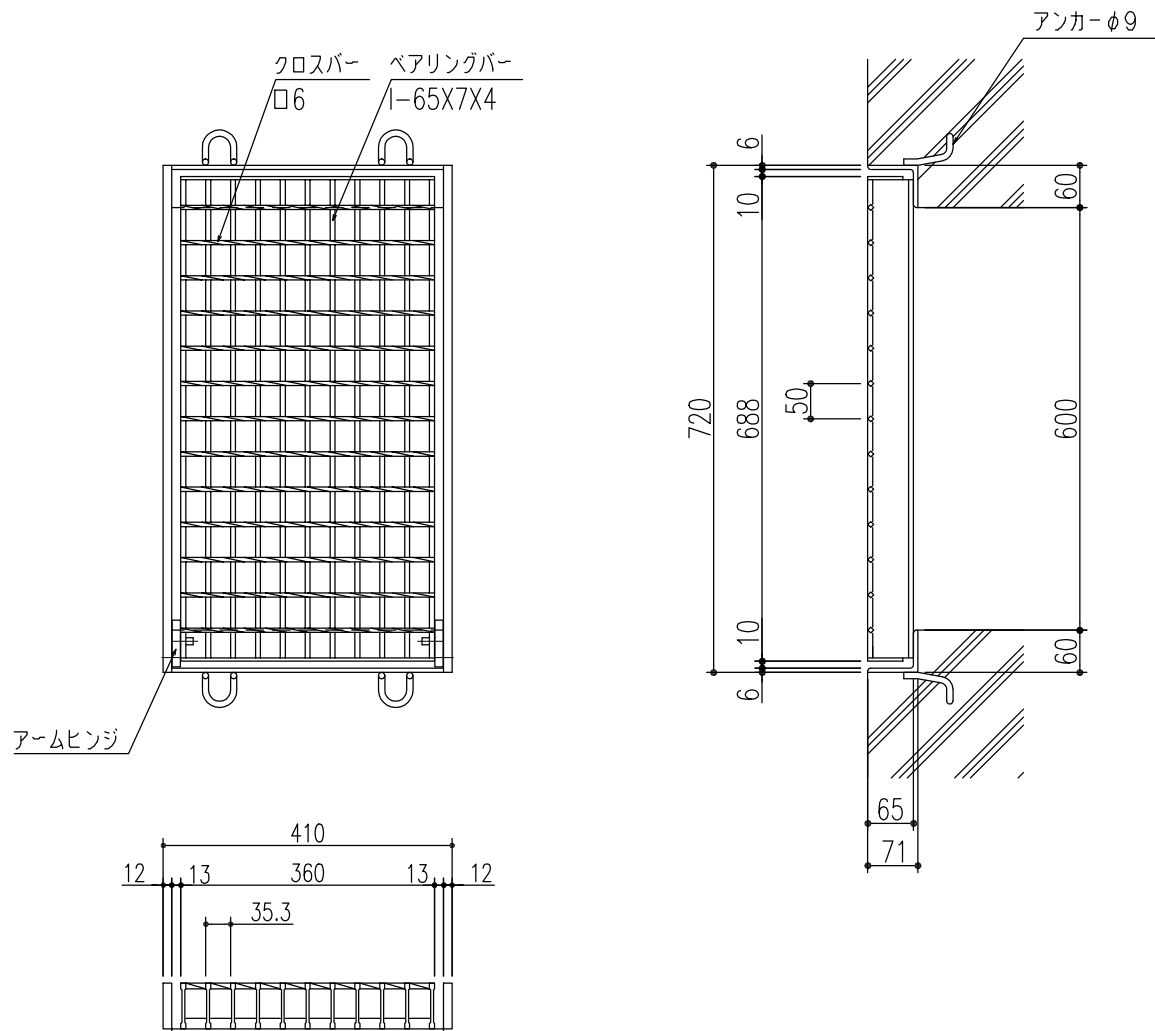
ベアリングバー 詳細図
